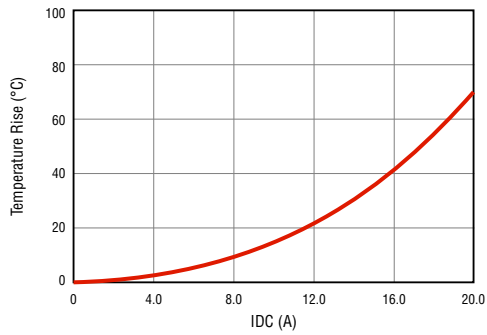
SRF1206A-701Y
