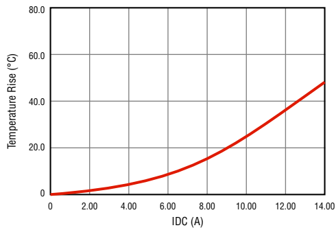
SRF1206A-501Y
