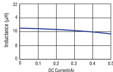
SRN2010TA-180M
