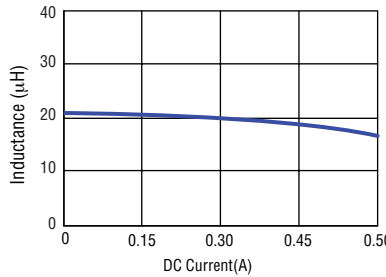
SRN3015TA-220M
