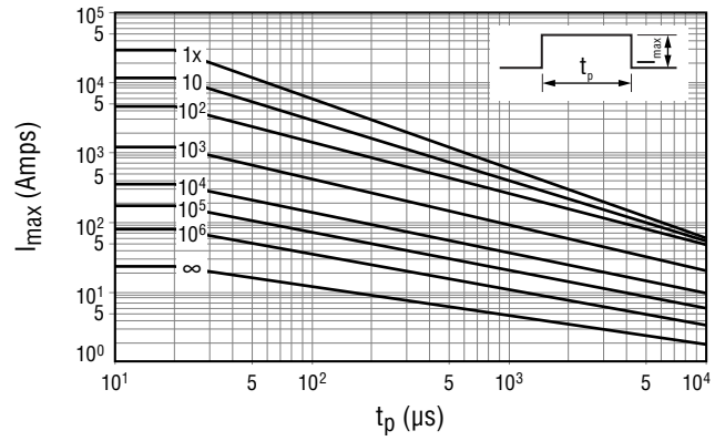
Model Size 32 - (ZOVR 60 K 32 ~ ZOVR 680 K 32)
