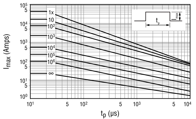
Model Size 40 - (ZOVR 60 K 40 ~ ZOVR 680 K 40)
